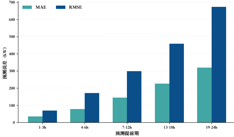
图 10 附件 3 官方光伏预测误差随提前期的变化
