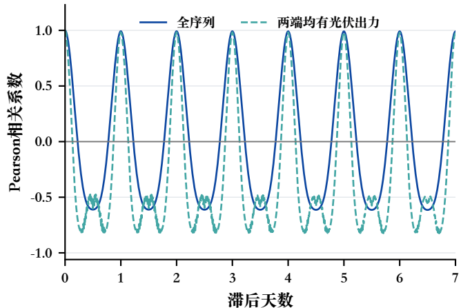
b 完整日、周时滞相关
