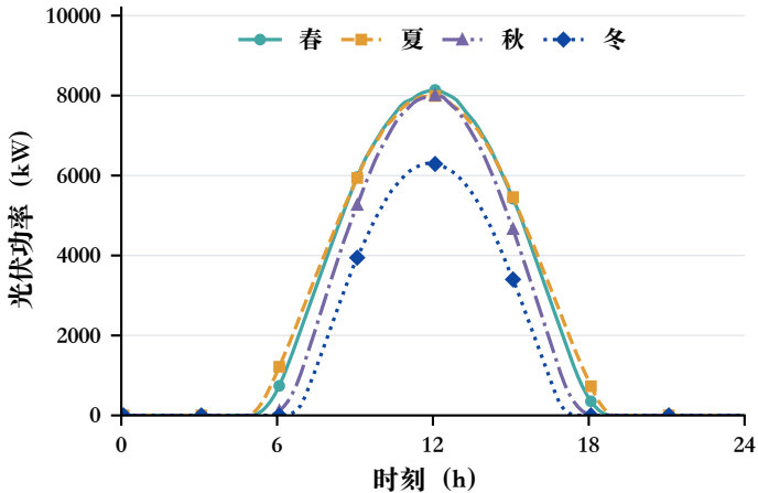
a 各季节平均光伏日轮廓
