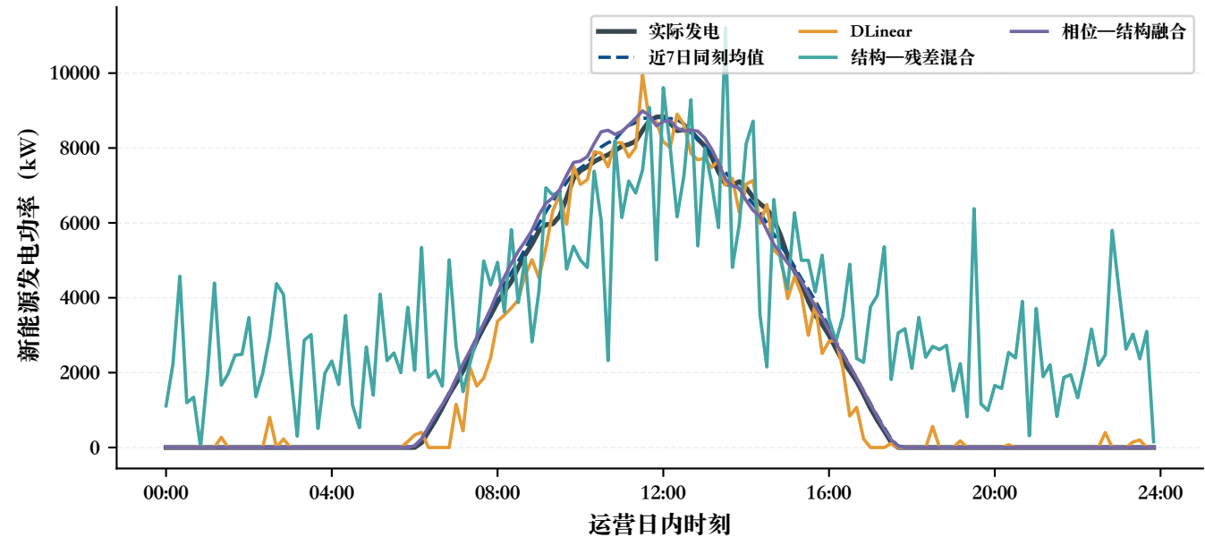
典型日预测轨迹 (2025-10-04)
