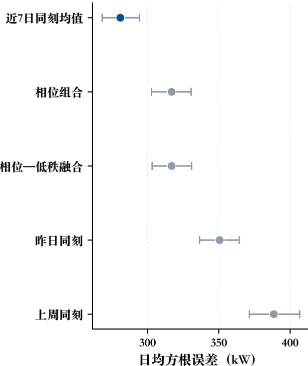
相位类方法与融合
