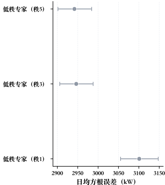
Hankel低秩解析外推
