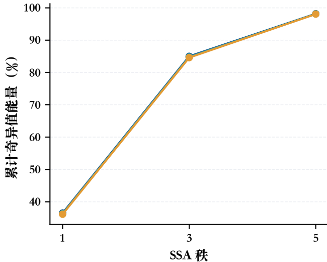
b 低秩能量保留率
