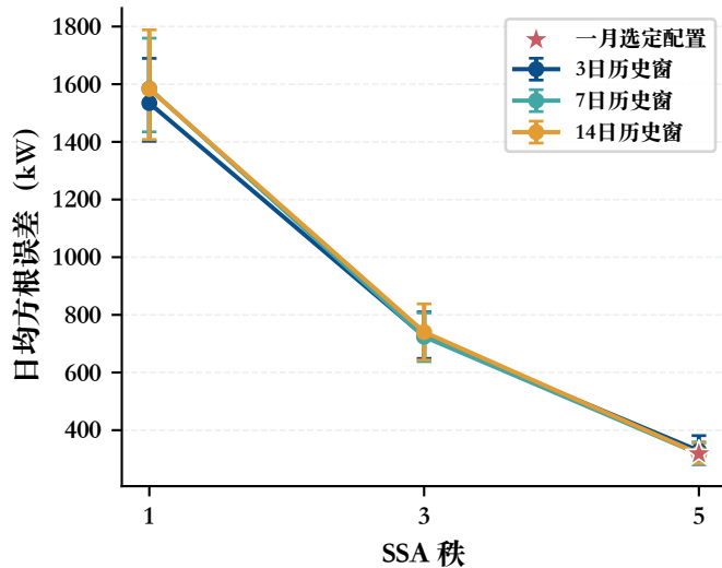
a 一月滚动验证误差
