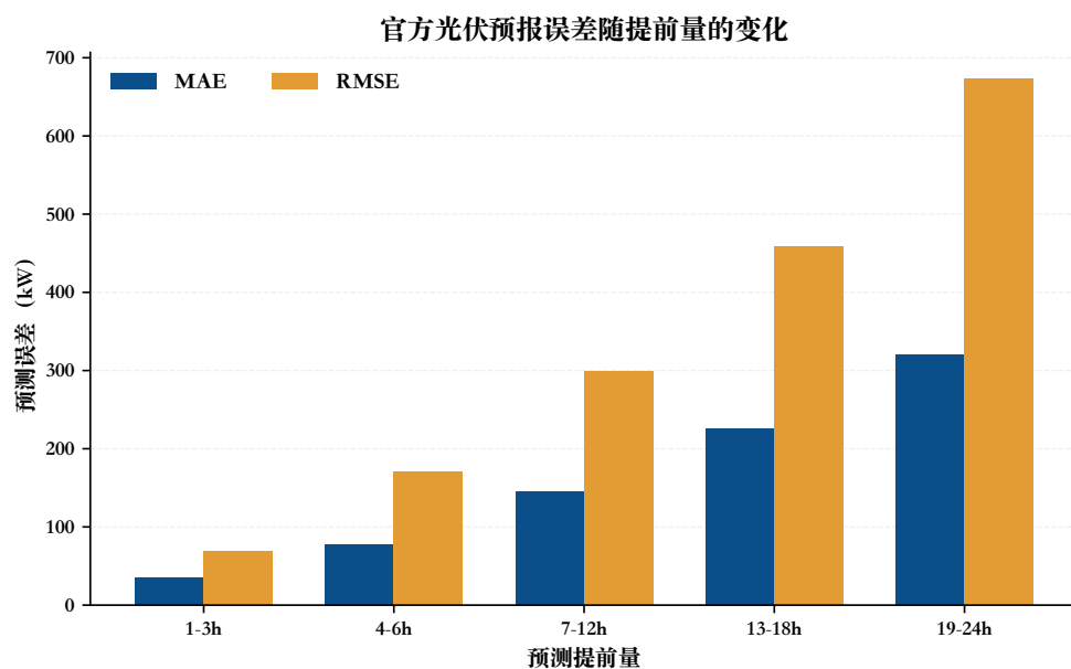
图 4 官方光伏预报在不同预测提前量下的 MAE 与 RMSE
