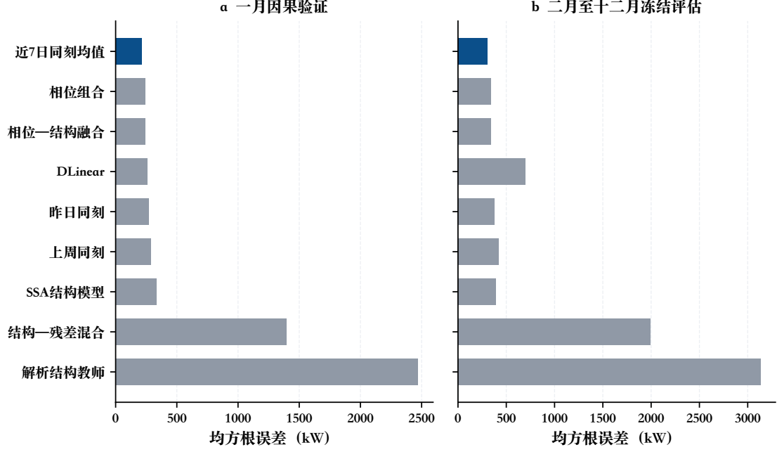
图 9 候选模型在一月统一验证期与 2–12 月冻结评价期的 RMSE。深蓝色表示仅依据一月验证选定的正式模型；右图不参与模型选择。
