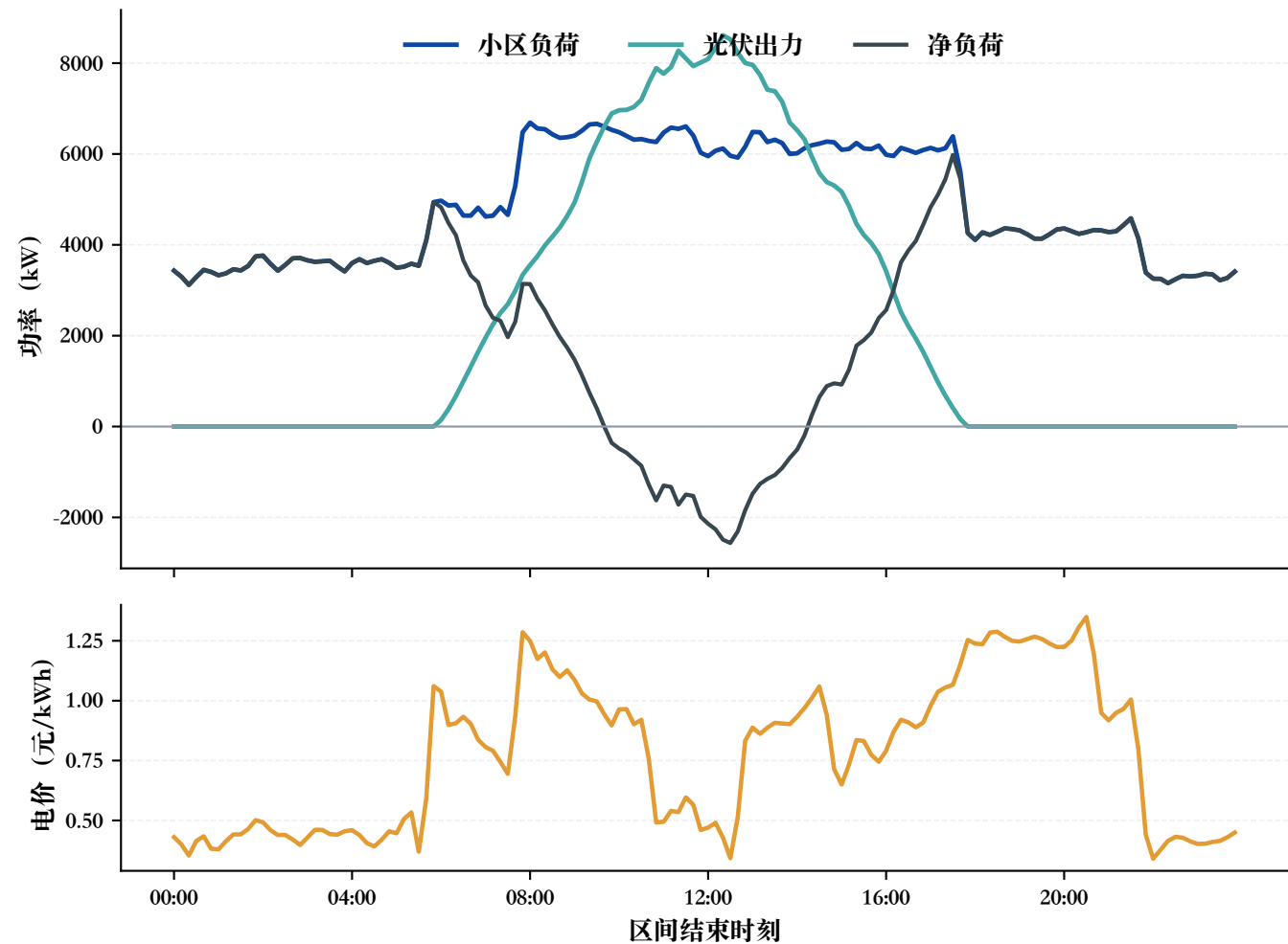
代表日负荷—光伏—净负荷结构 (2025-03-19)
