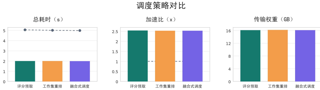
图 5.4 不同调度配置的真实 offload 调度对比
