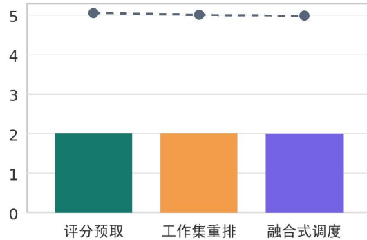
总耗时 (s)
