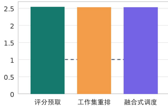
加速比 (x)
