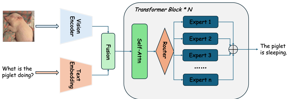
图 1.1 VL-MoE 模型的一般推理链路及专家路由示意图
