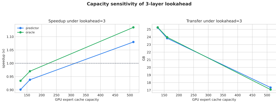
图 5.3 lookahead=3 下不同缓存容量的收益变化
