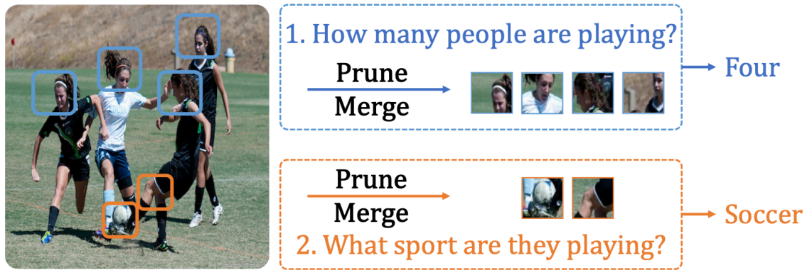
图 3.1 不同文本问题下语义相关视觉 Token 的保留重点示意图
