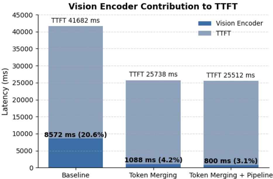
图 5.1 Visual Encoder 优化对 TTFT 的影响
