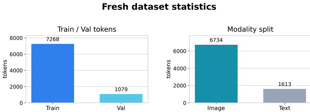
图 4.3 训练数据规模与模态分布统计
