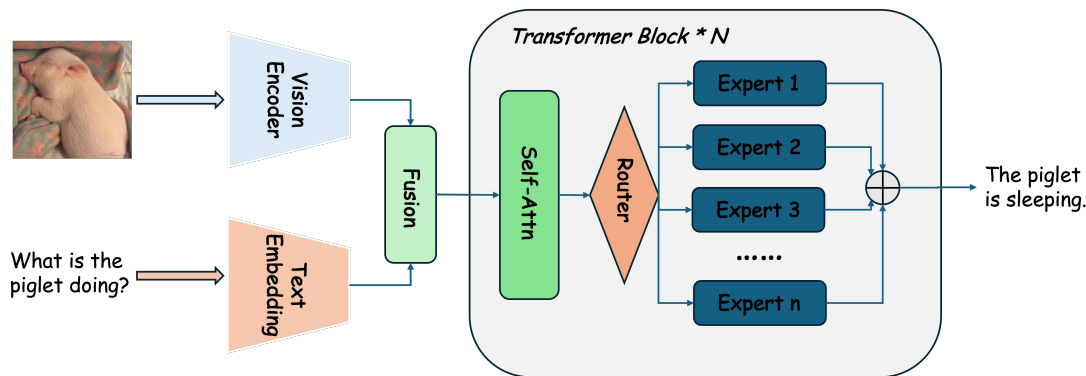
图 1.1 VL-MoE 模型的一般推理链路与专家路由示意图
