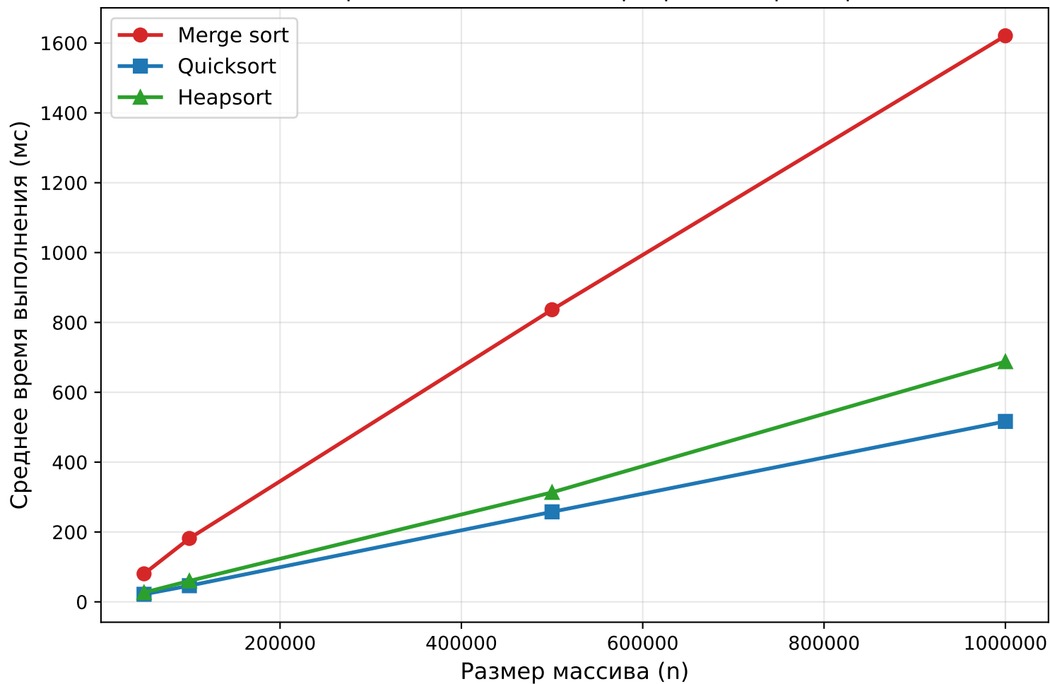
Зависимость времени выполнения сортировок от размера массива
