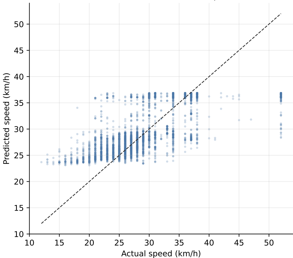
LSTM Actual vs Predicted Speed
