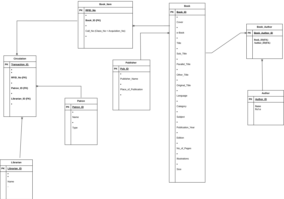
ER Diagram
