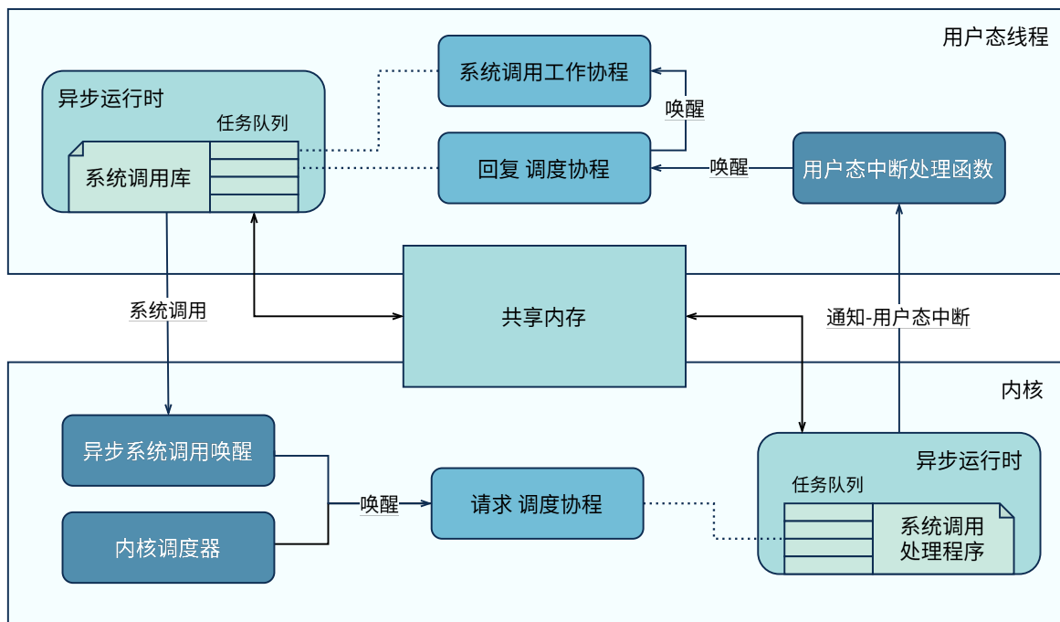
图 3-1 ReL4 中异步系统调用流程
