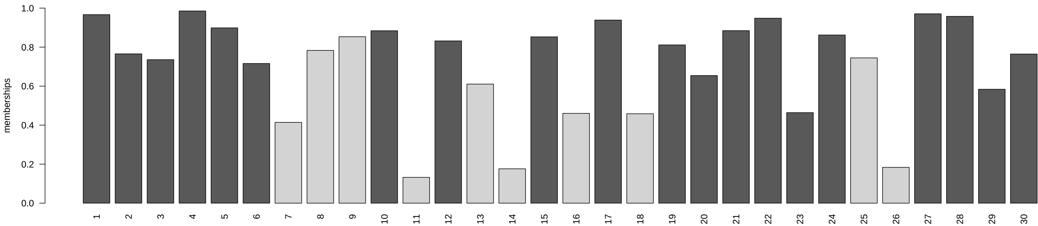
Motif 2
