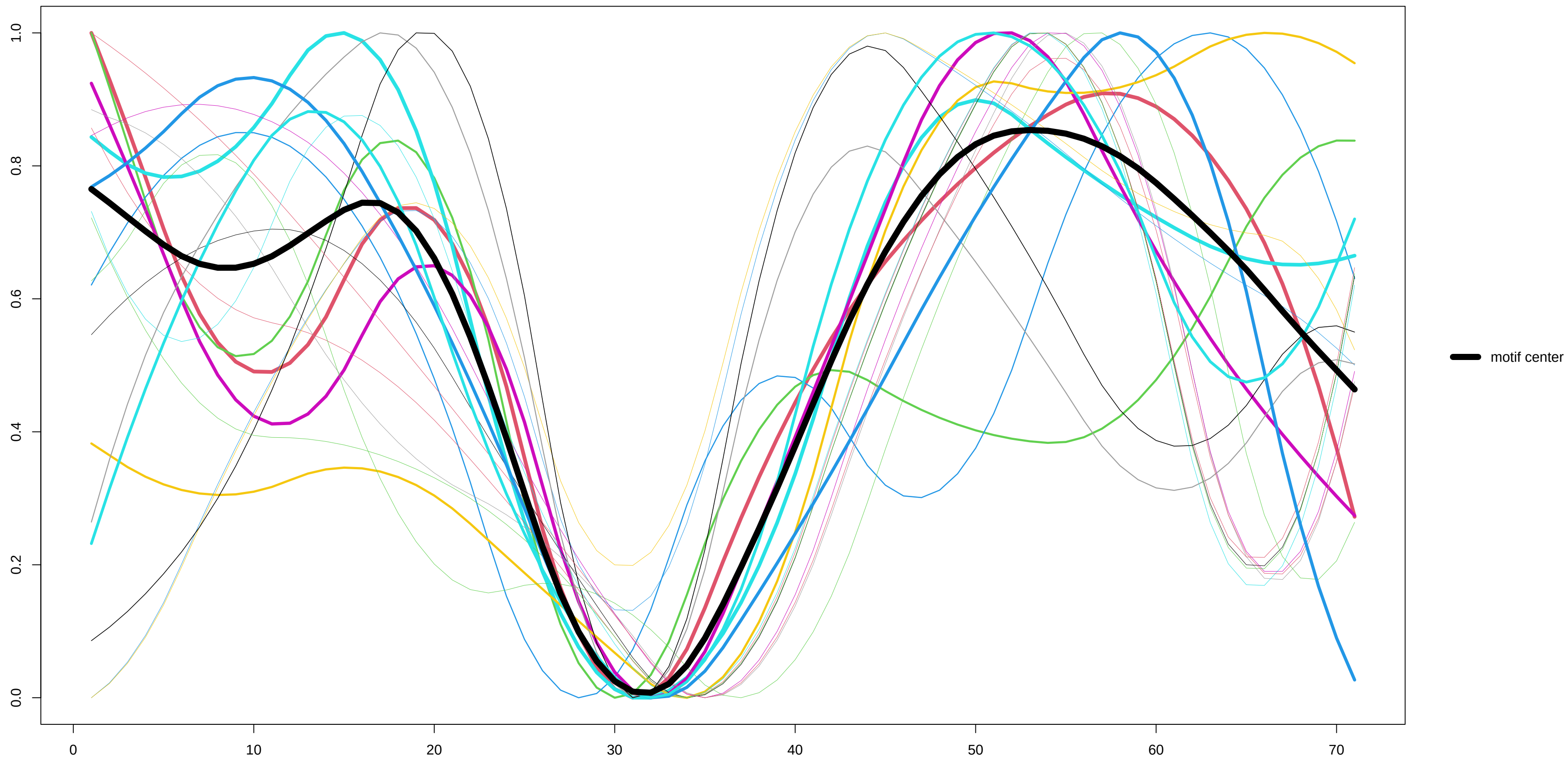
Motif 1 –
