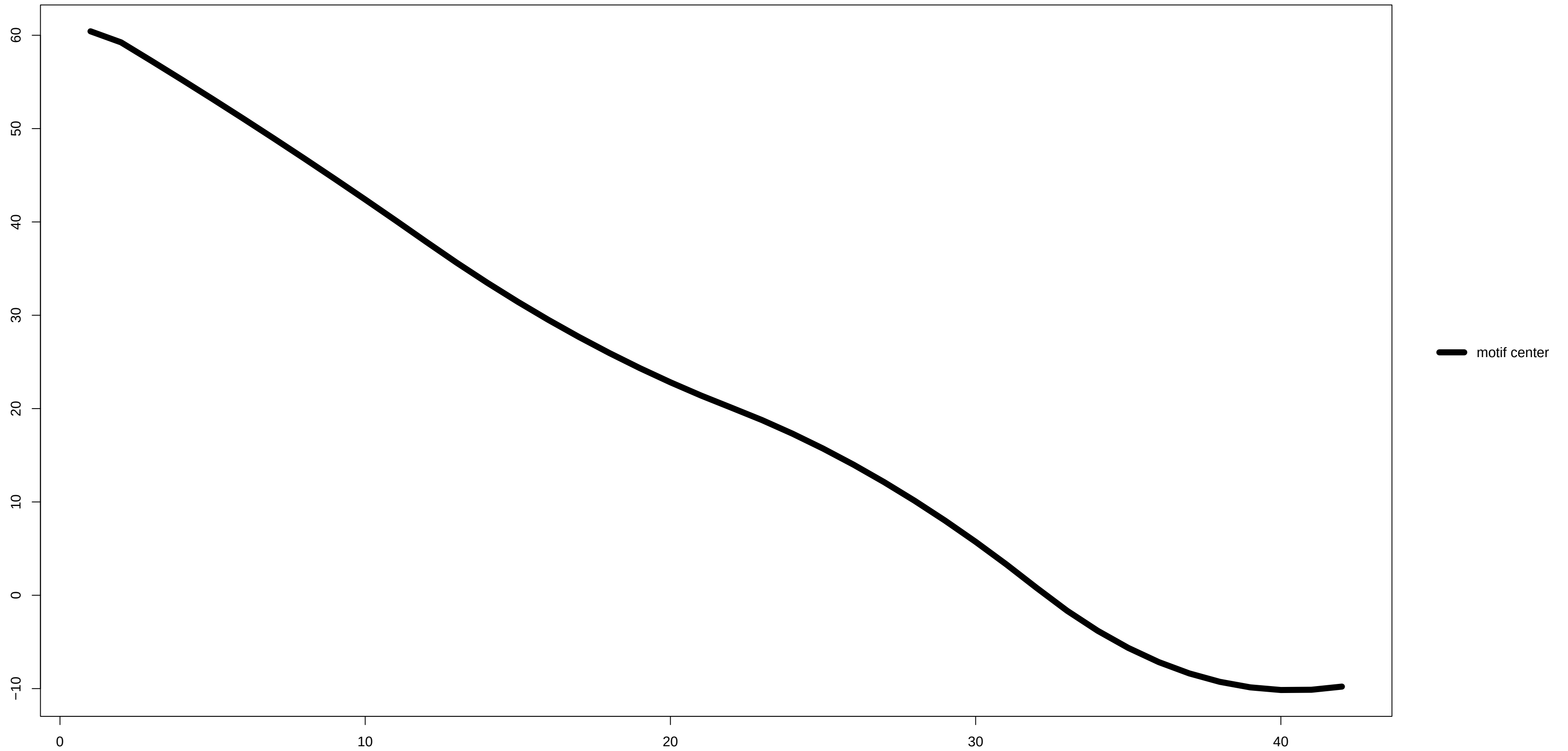
Motif 1 –
