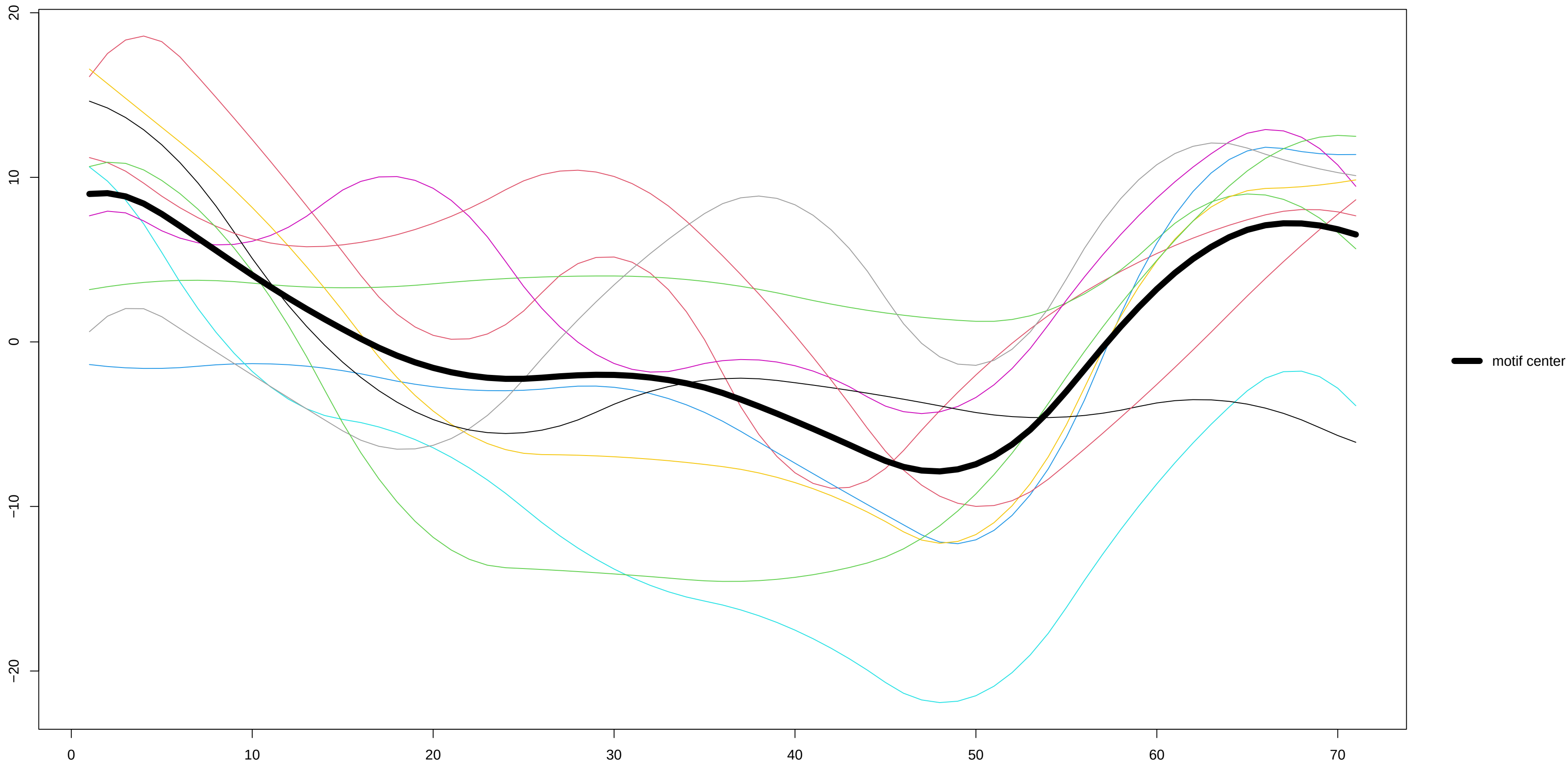
Motif 3 –
