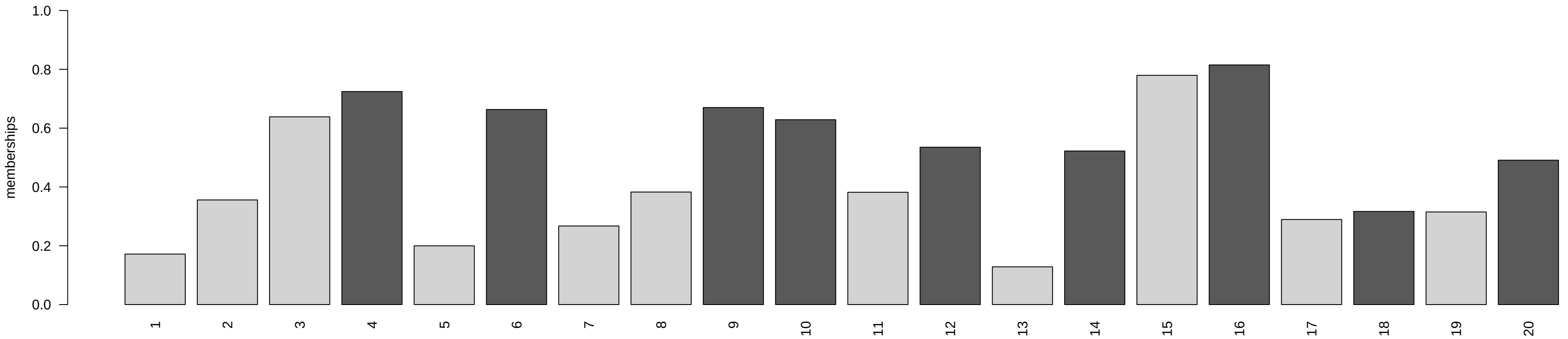
Motif 2
