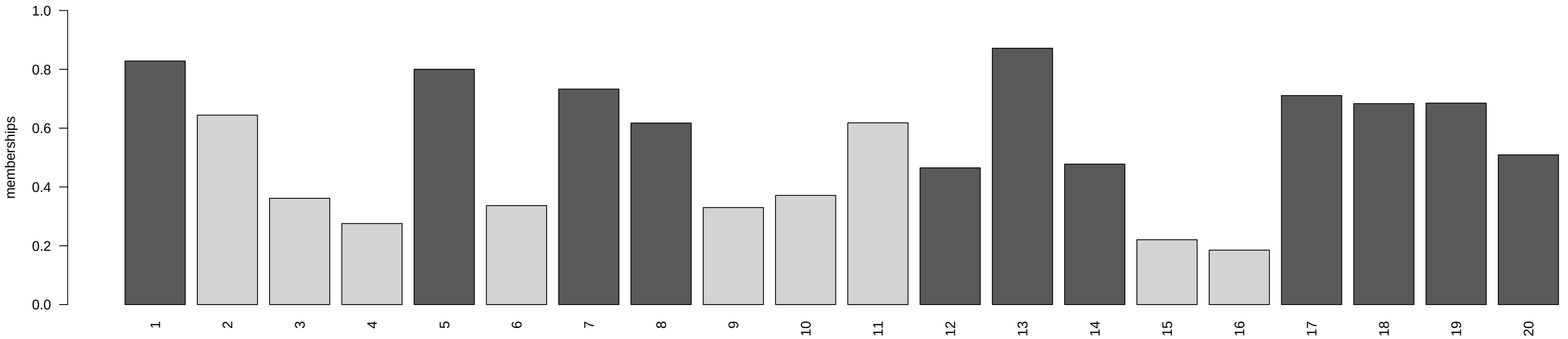
Motif 1
