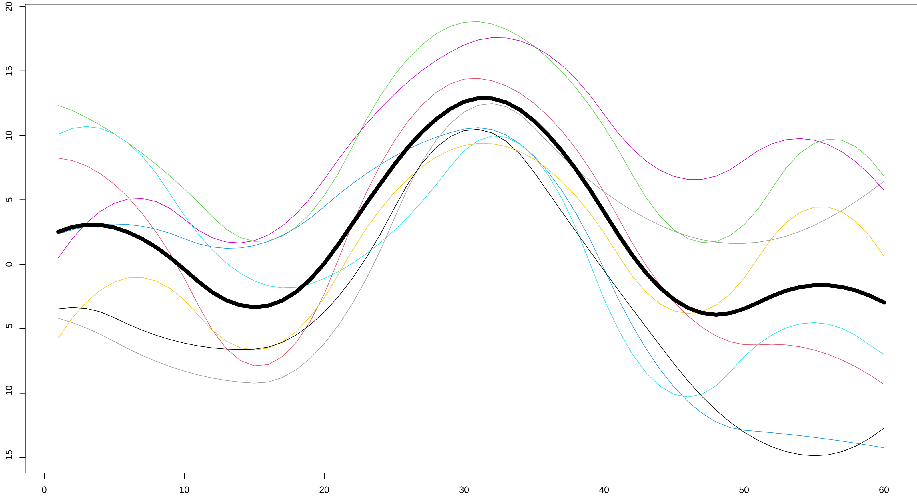
Motif 3 –
