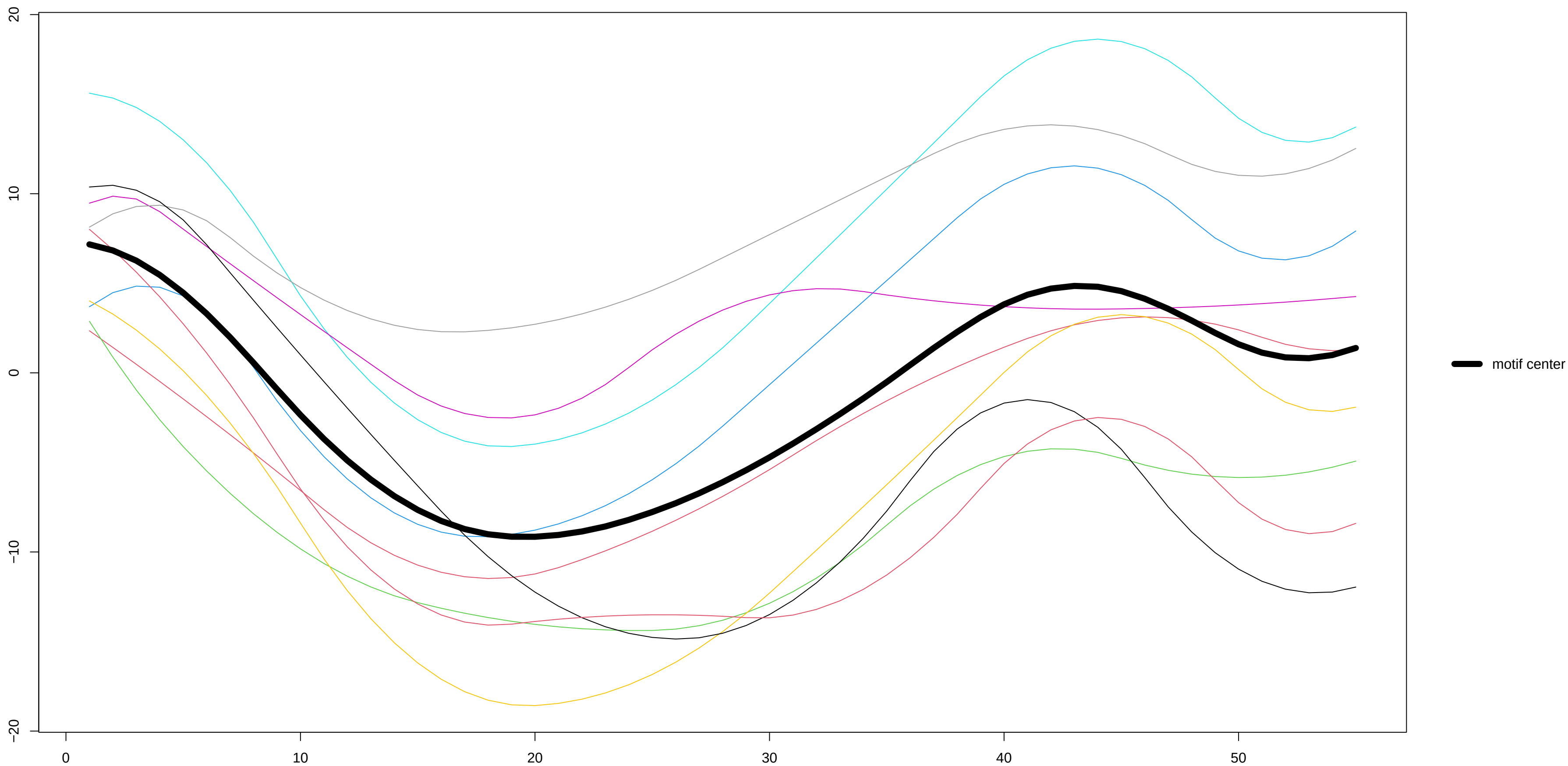
Motif 1 –
