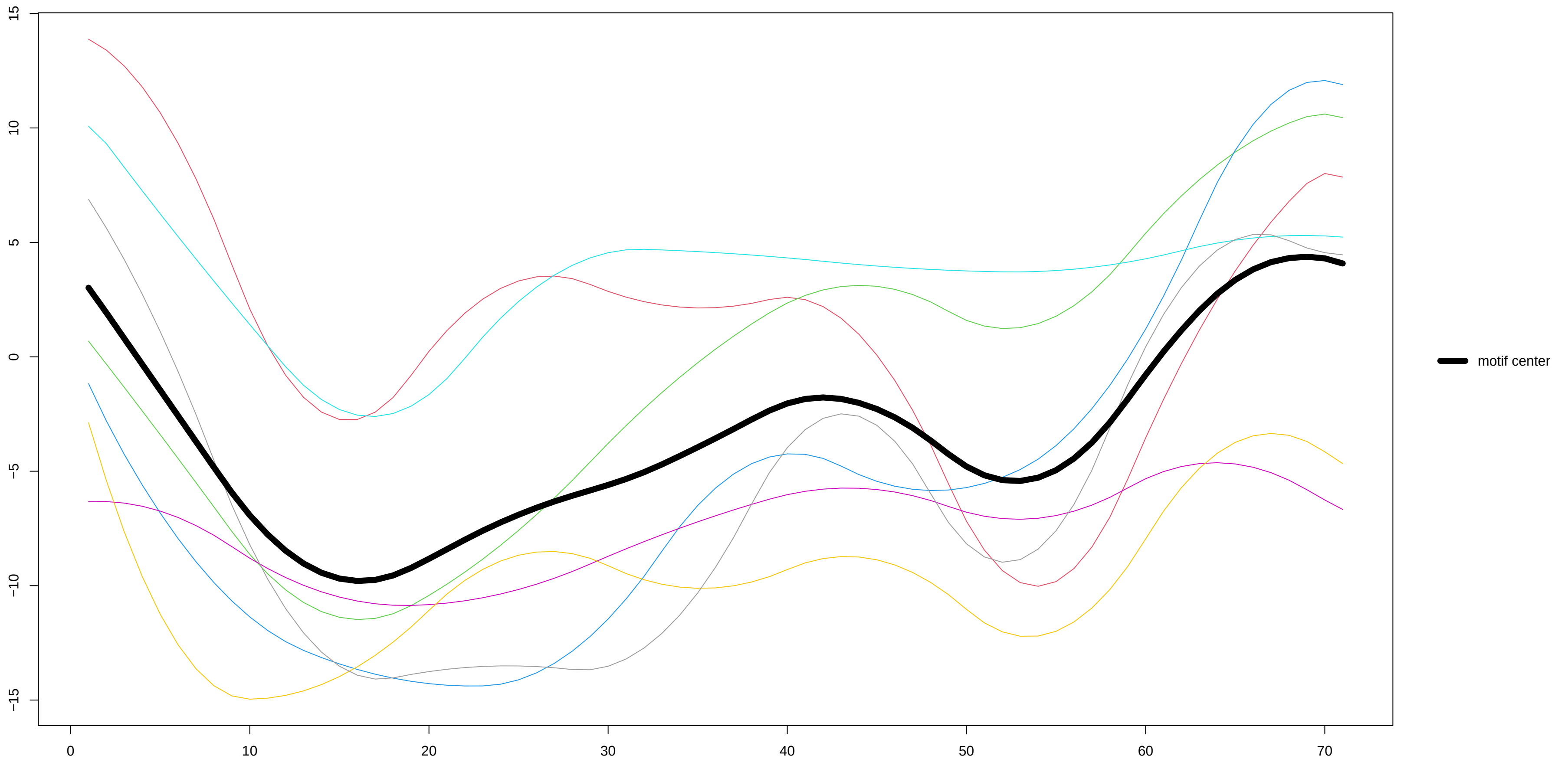
Motif 3 –
