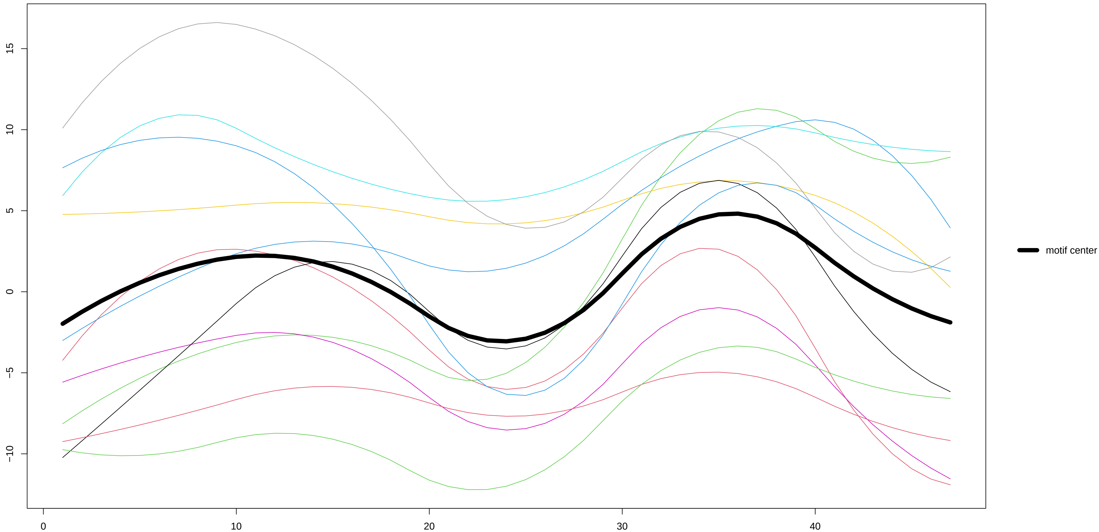
Motif 2 –
