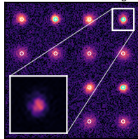
min.-var. branching
