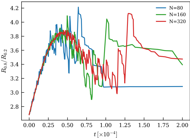
(d) core-halo separation
