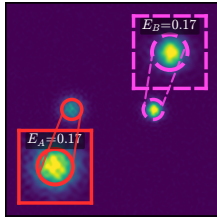
min.-var. branching
