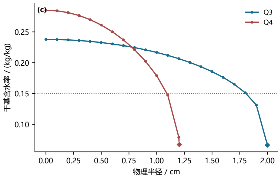
同一 24 h 径向剖面
