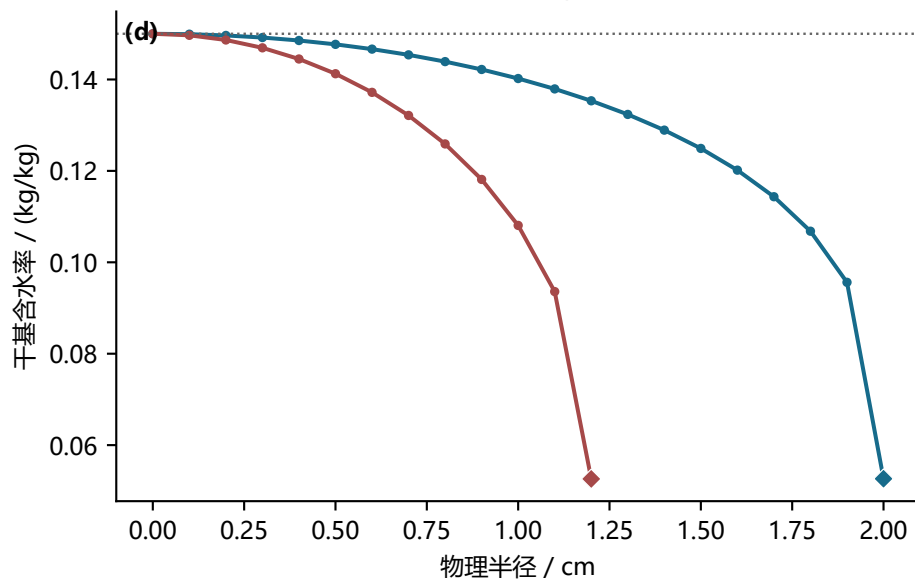
各自全域达标时径向剖面
