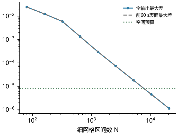
相邻网格含水率差 / ( \text{kg}/\text{kg} )
