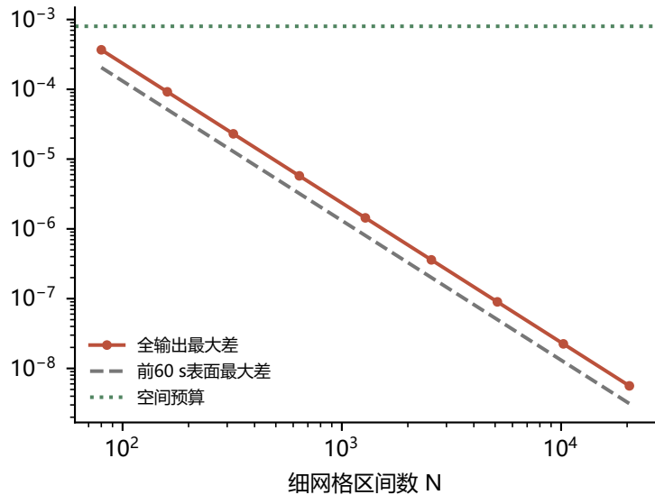
相邻网格温度差 / ^{\circ}\text{C}
