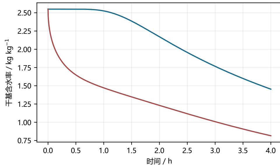
含水率早期细节 (0-4 h)
