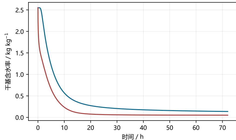
含水率全程 (0-72 h)
