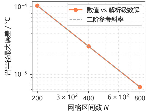
(a) 温度 (附录2 常物性, t = 100 s)
