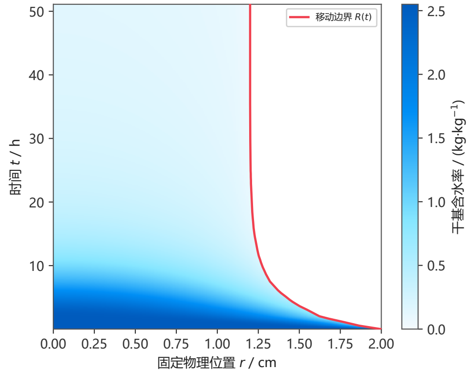
(a) 含水率场与移动边界 (域外留白、严格裁切)
