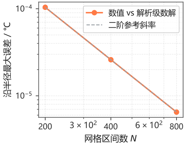
(a) 温度 (附录2 常物性, t = 100 s)
