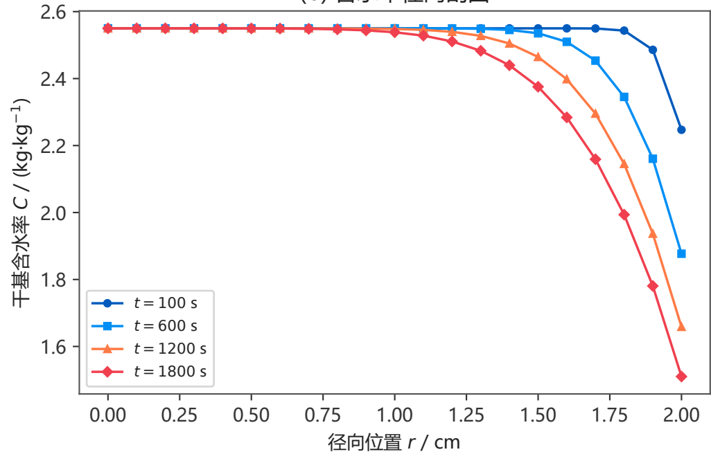
(b) 含水率径向剖面
