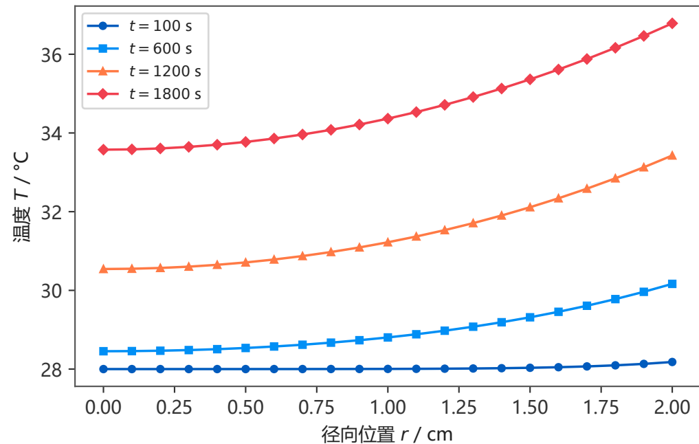
(a) 温度径向剖面
