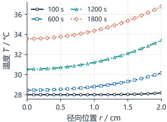
(a) 温度径向剖面
