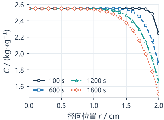
(b) 含水率径向剖面
