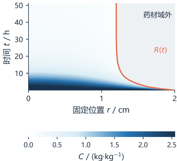
(a) 含水率场与收缩边界
