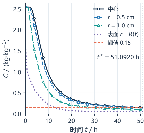
(b) 固定位置与表面时程
