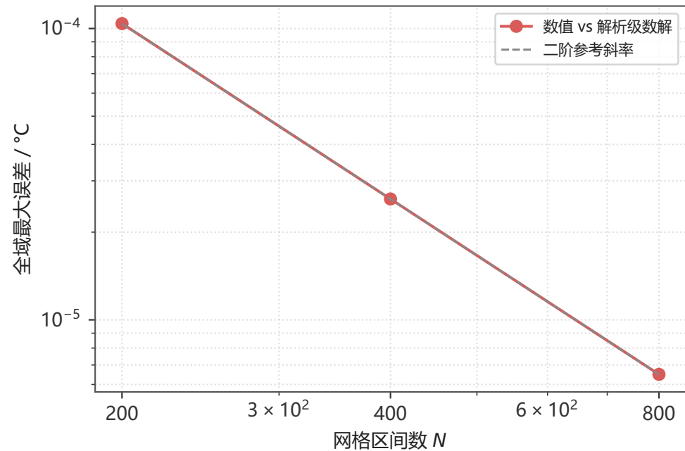
(a) 温度 (附录2 常物性辅助问题)
