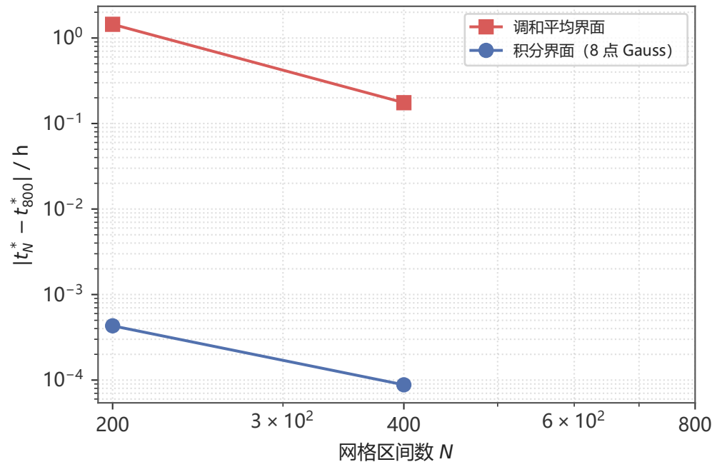
(b) 相对最细网格的收敛 (对数)
