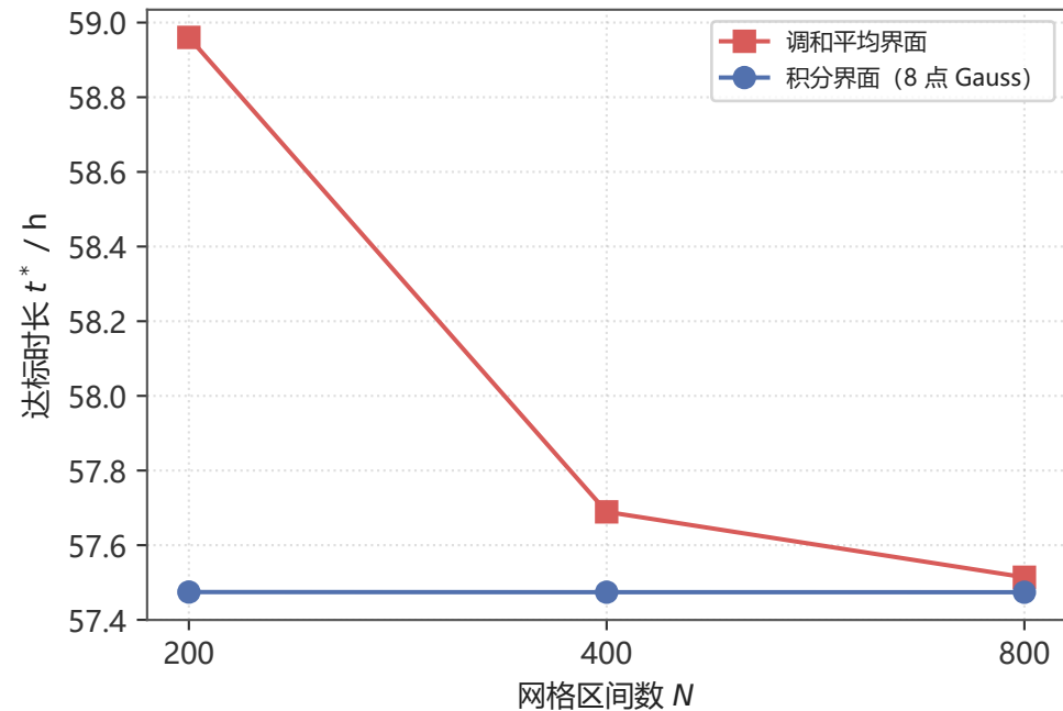
(a) 达标时长随网格加密
