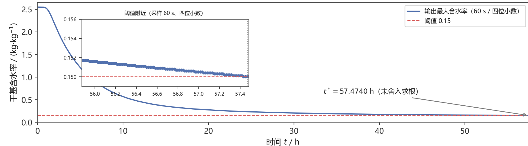
(c) 输出最大含水率随时间下降; 阈值附近仅示采样分辨率
