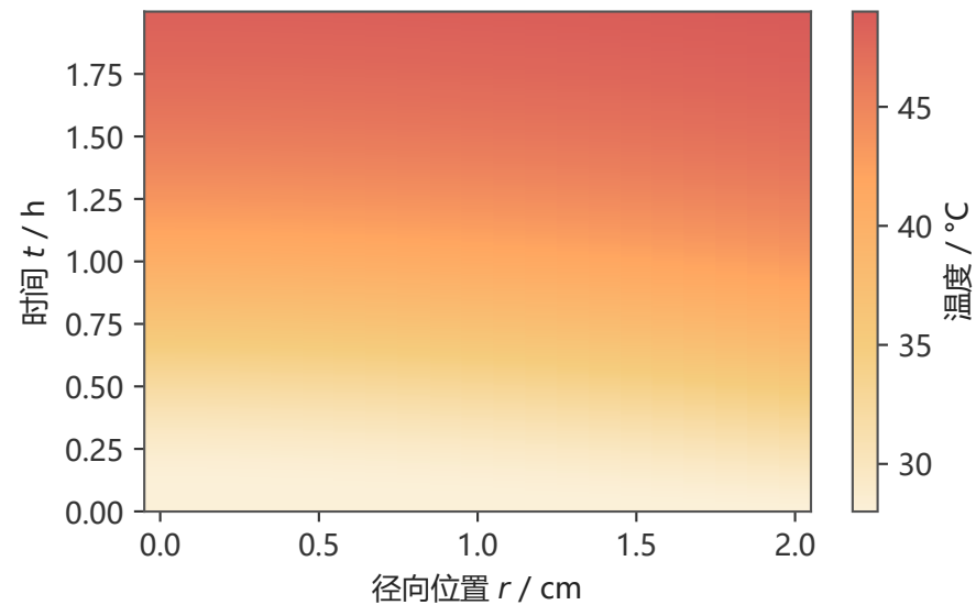
(a) 温度场演化 (0-2 h, 附录3)
