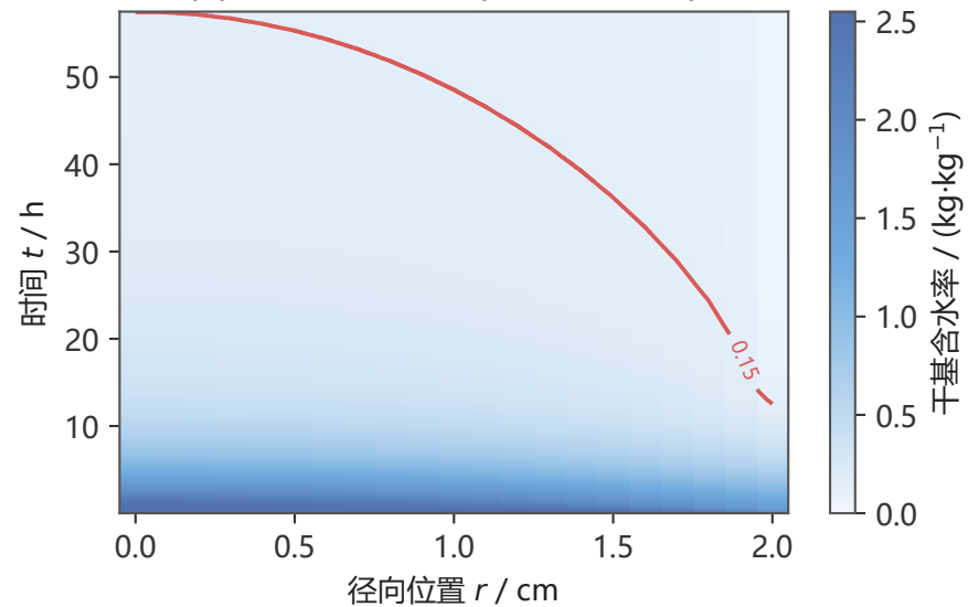
(b) 含水率场演化 (全程, 附录3)
