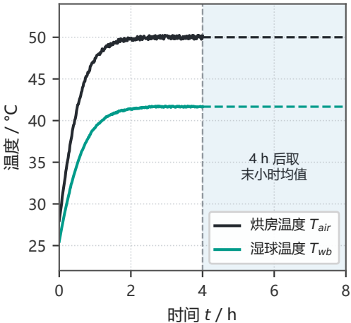
(a) 烘房温度与湿球温度
