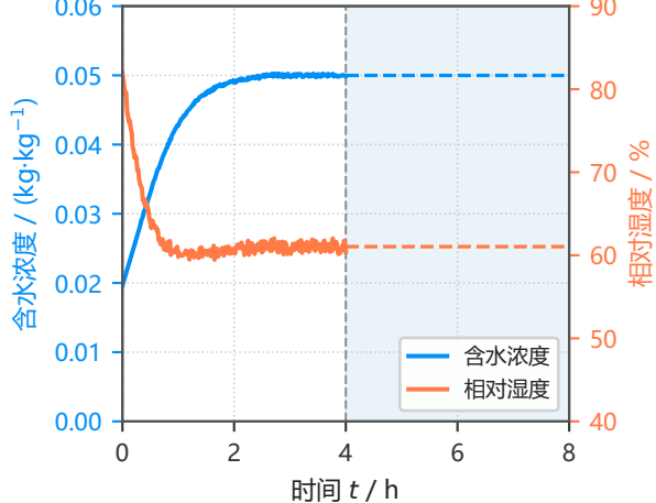
(b) 含水浓度与相对湿度
