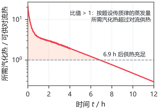
(c) 题设模型的表面能量核算
