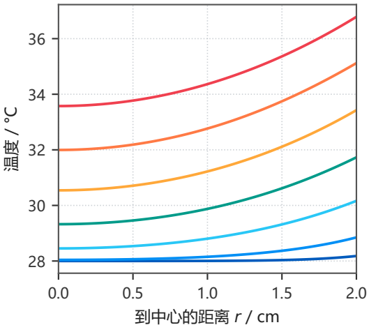
(a) 温度剖面
