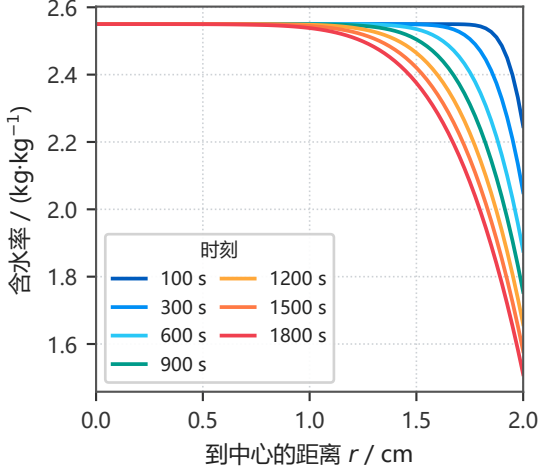
(b) 含水率剖面
