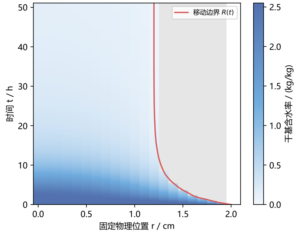
(a) 含水率场与移动边界 (域外淡灰)
