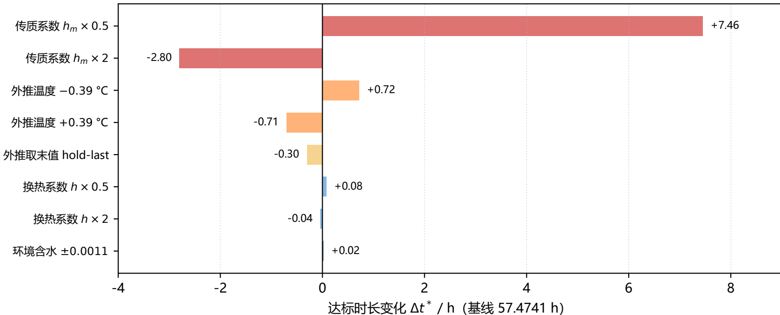
参数扰动对达标时长的影响 (问题二/三, 人为扰动范围内)
