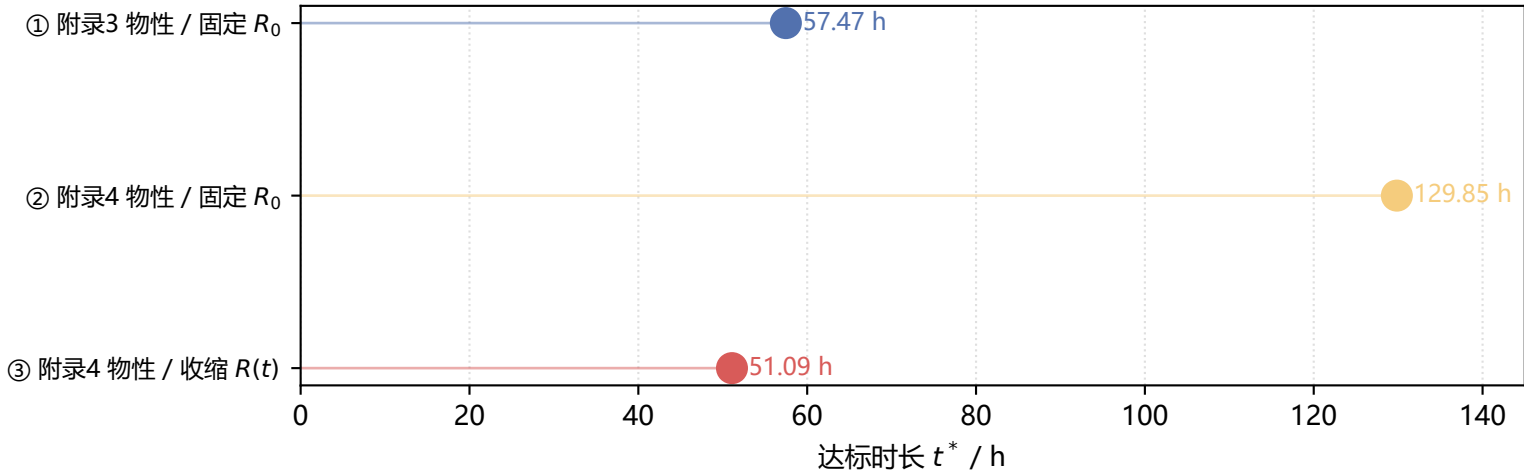
物性变化与尺寸收缩对达标时长的相反作用
