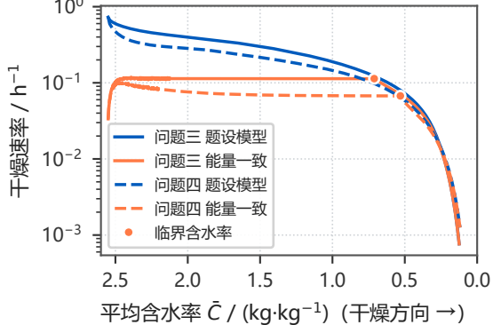
(b) 干燥速率曲线
