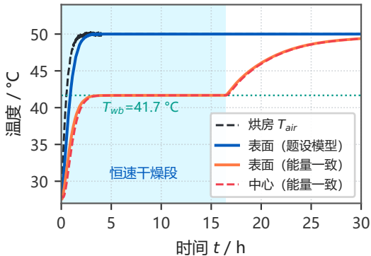
(a) 问题三物料温度
