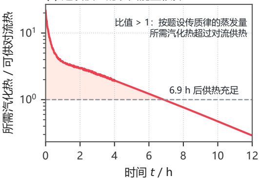
(c) 题设模型的表面能量核算
