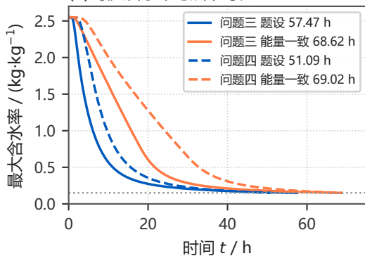
(d) 最大含水率与烘干时长
