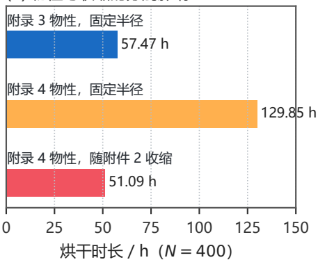
(d) 物性与收缩的分别影响
