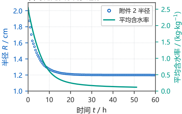
(c) 收缩与失水同步进行
