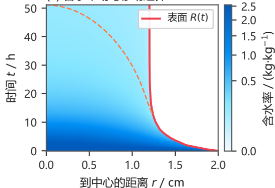
(a) 含水率场与移动边界
