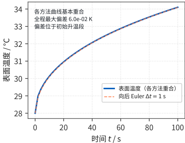
(a) 表面温度时程
