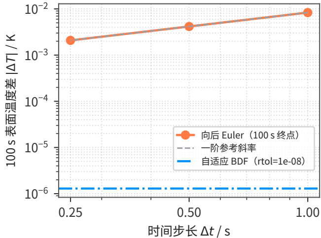
(b) 相对紧容差 BDF 参考的差异
