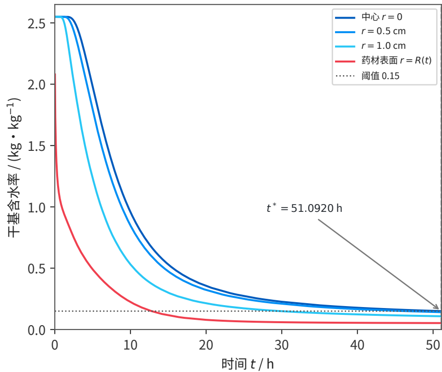
(b) 固定位置与表面含水率时程
