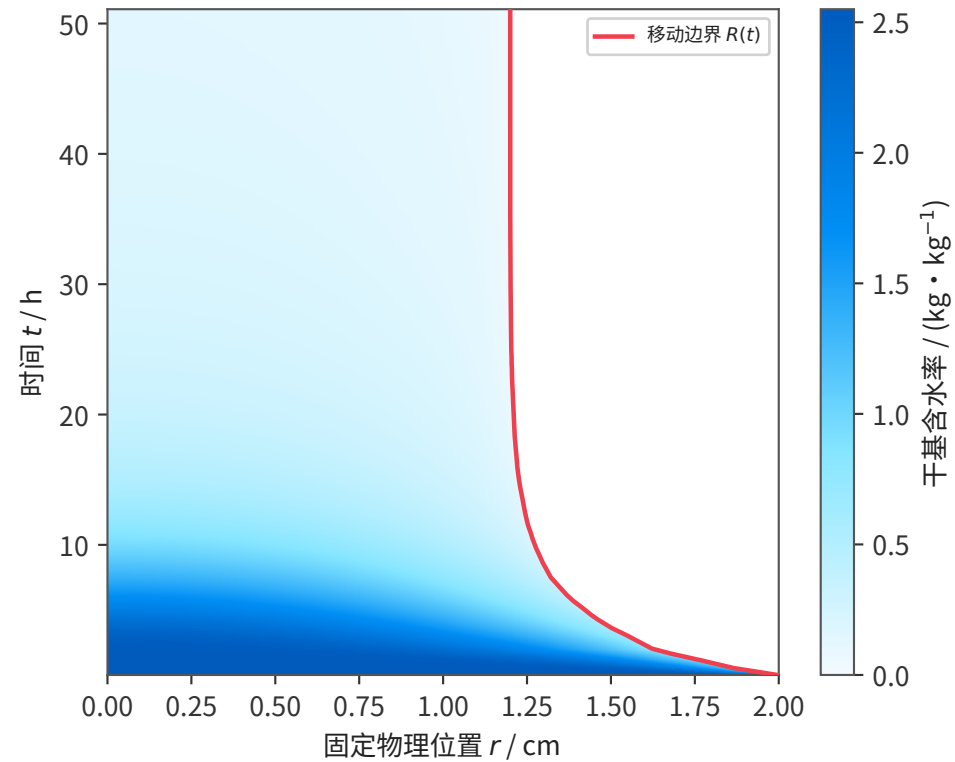
(a) 含水率场与移动边界
